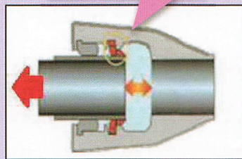
耐震継手管の構造（イメージ）
